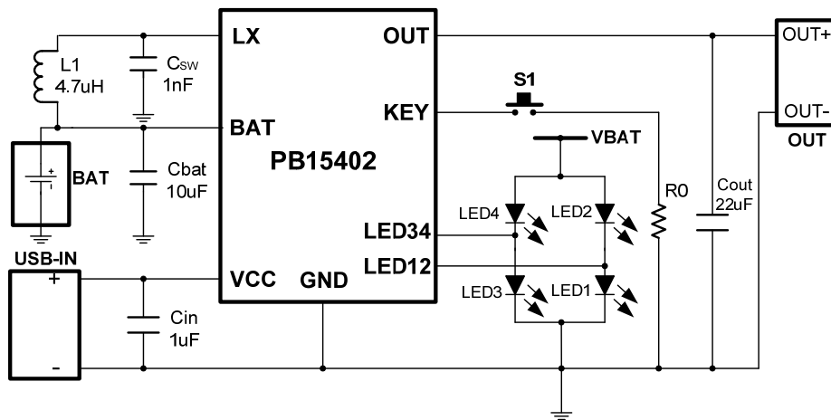
图 1. PB15402 典型应用
