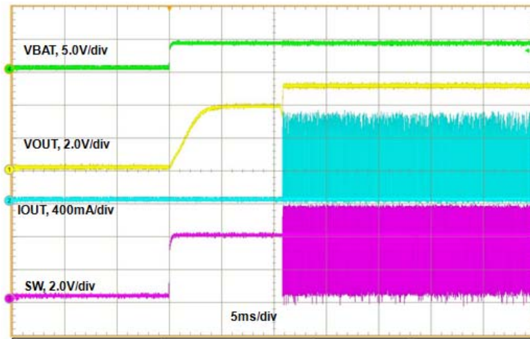
升压启动波形, R_{OUT}=100\Omega
