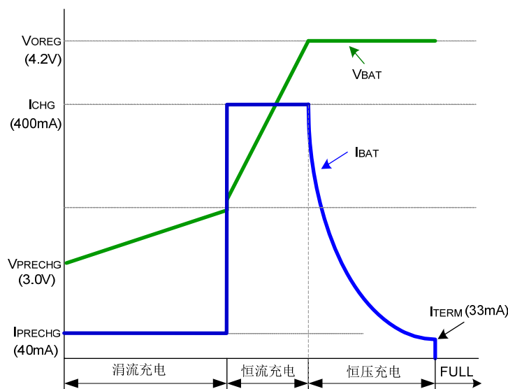
图 3. PB15402 充电曲线
