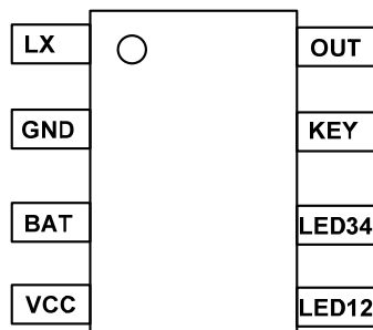
图 2. PB15402 SOP8 封装顶视图
