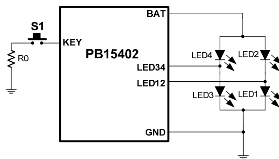
图 4. KEY 键连接示意图
