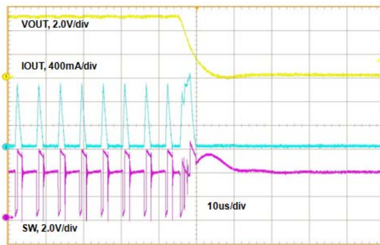
VOUT 短路响应波形, V_{BAT}=3.8V
